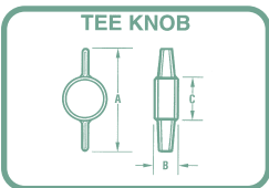
TEE KNOB
